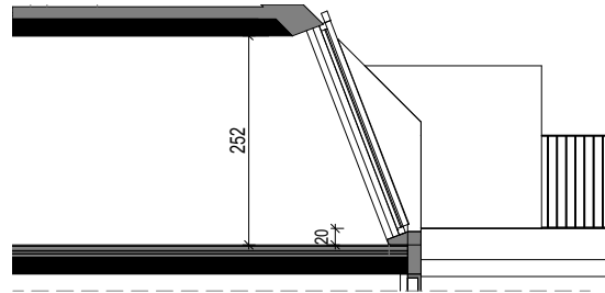
Schnitt 44.A
