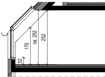
Schnitt 44.B
